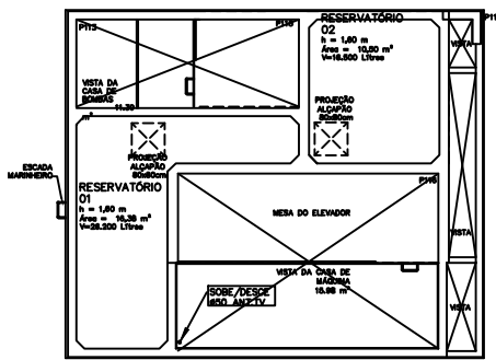
PLANTA BAIXA CX D'AGUA ESCALA 1:50
