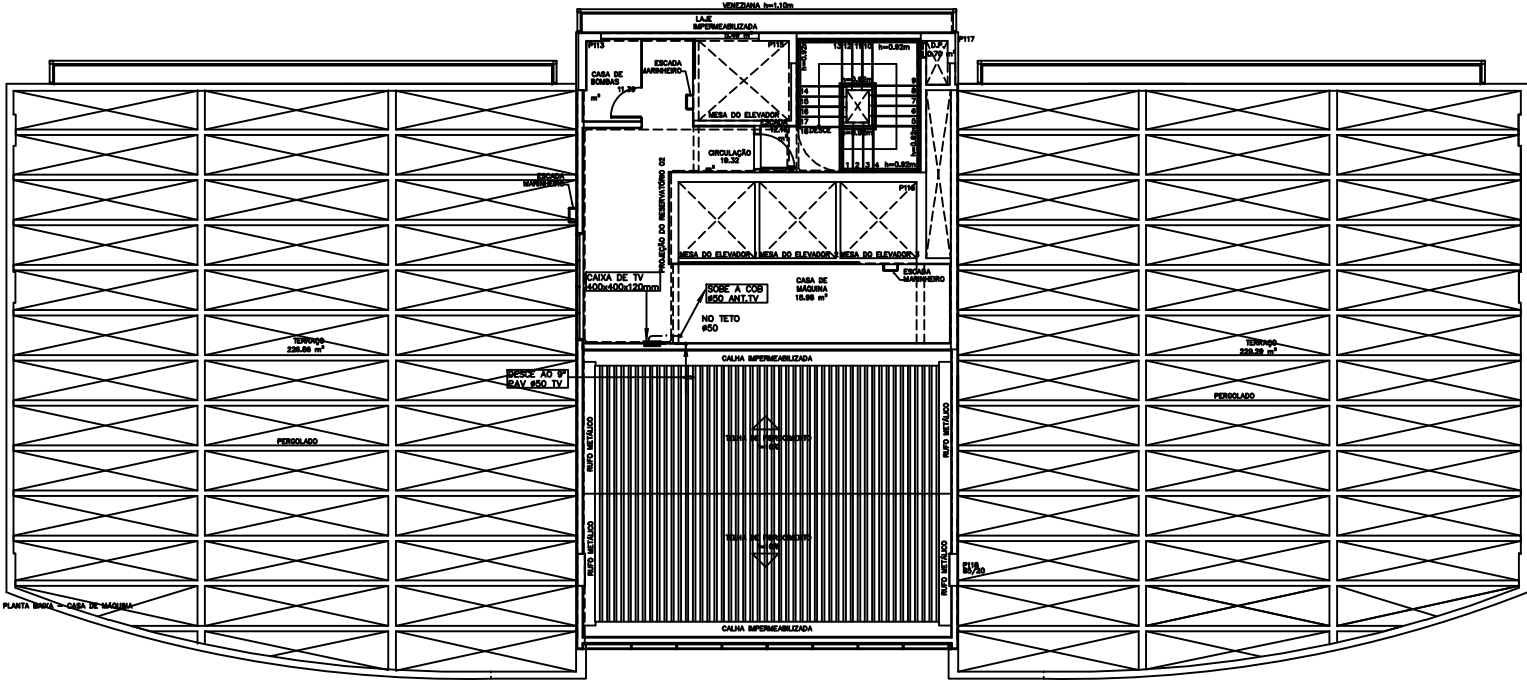
PLANTA BAIXA COBERTURA – BLOCO "A" ESCALA 1:100
