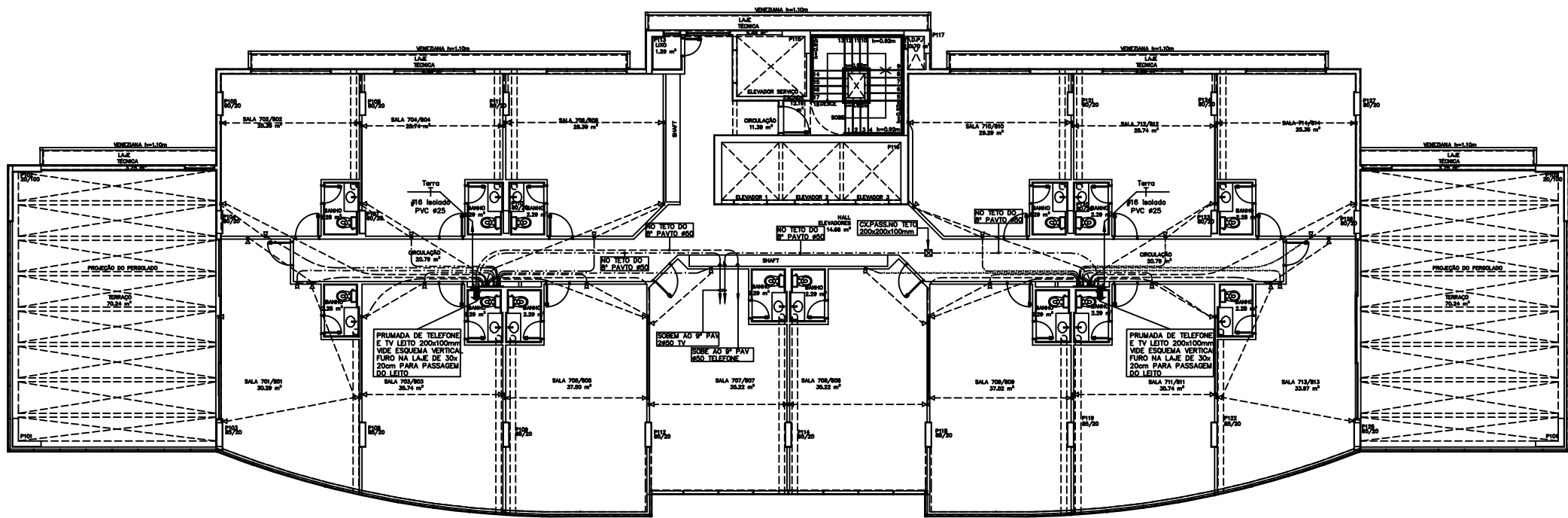
PLANTA BAIXA 7º E 8º PAVIMENTO – BLOCO "A" COMERCIAL ESCALA 1:100
