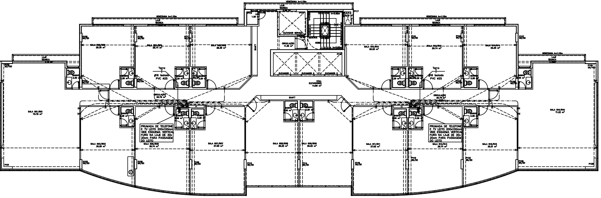
PLANTA BAIXA PAVIMENTO 5º AO 6º – BLOCO "A" COMERCIAL ESCALA 1:100
