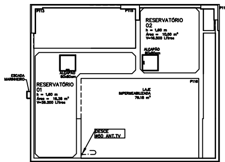
PLANTA BAIXA COBERTURA CS.MAQ. ESCALA 1:50
