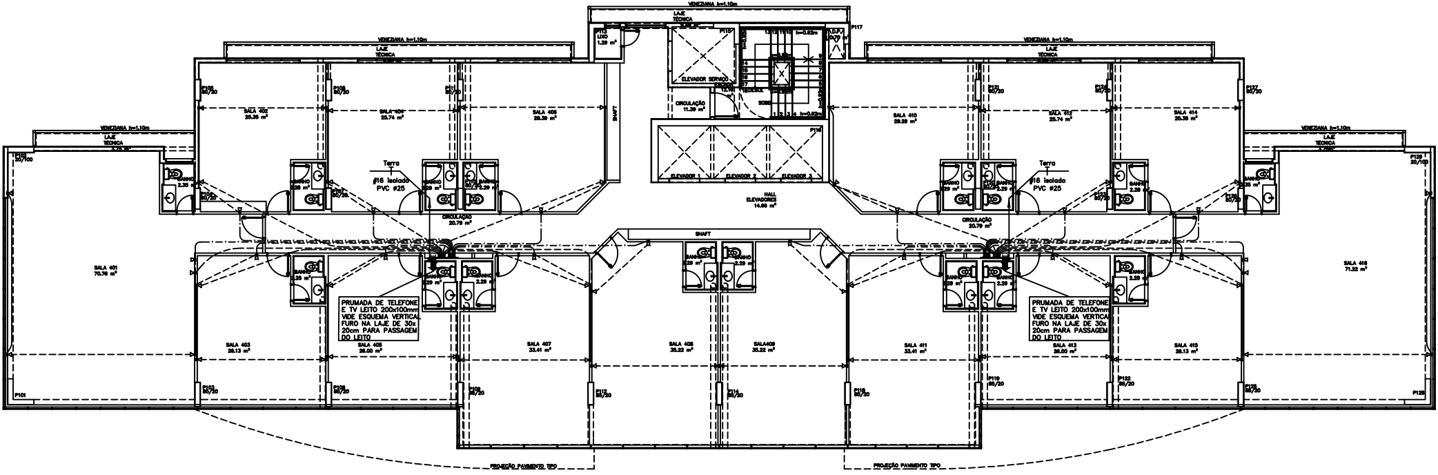
PLANTA BAIXA PAVIMENTO 4º – BLOCO "A" COMERCIAL ESCALA 1:100
